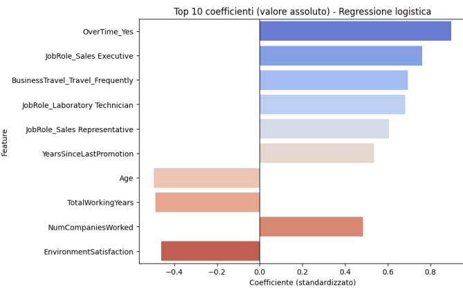
Figura 5. I 10 coefficienti (in valore assoluto) più rilevanti della regressione logistica, su feature standardizzate (Fase 5).
