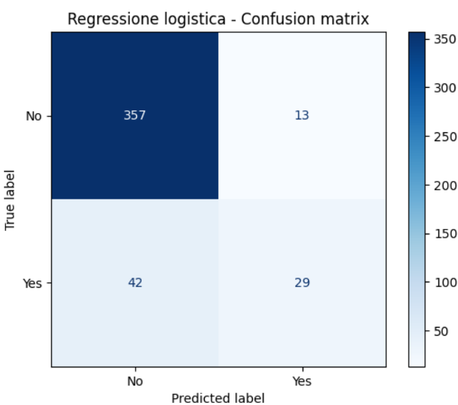
Figura 4. Matrice di confusione della regressione logistica sul test set (Fase 5).
